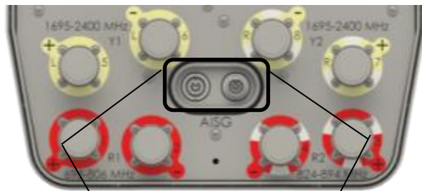
AISG I/O Configuration
